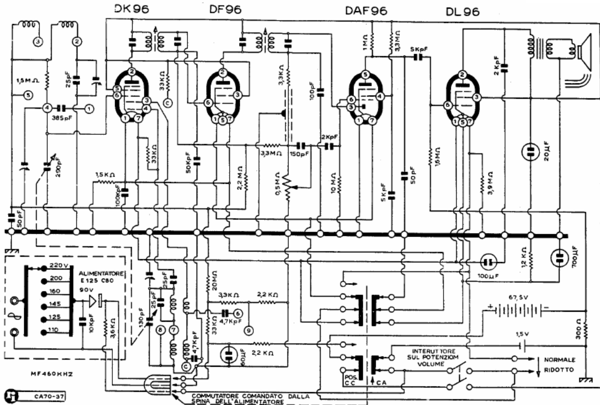
VEGA RADIO - TV - Mod. 426 IIª Serie
